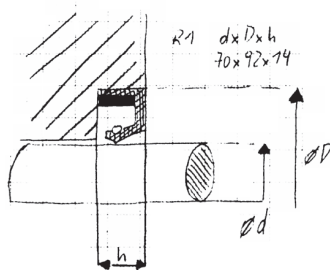
Rotordichtung/Wellendichtring
