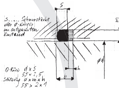
O-Ring / Stützring
