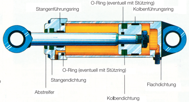
Abstreifer
