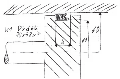
Kolbendichtung
