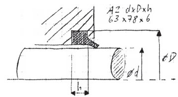
Abstreifer
