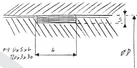
Führungsring
