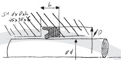
Stangendichtung
